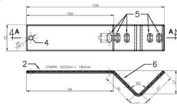
Figura 01 – Vista frontal e perfil – Medidas em mm.
