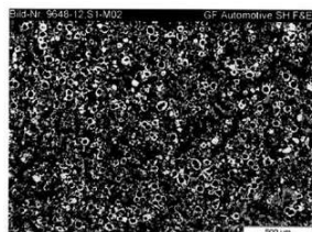
FIG. 1: Fotomicrografia da microestrutura da liga fundida nodular da invenção
