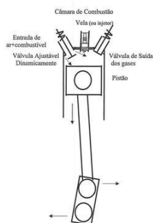
Figura 1 - Motor de Auto-Ignição por Controle da Entrada da Câmara
