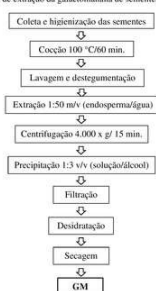
Figura 1 - Fluxograma de extração da galactomanana de sementes de Adenanthera pavonina .
