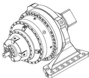
Fig. 1.7 Vista em perspectiva
