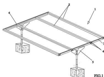
ESTRUTURA METÁLICA PARA COBERTURA SOLAR (71) SIGMA AÇO TUBOS E PERFILADOS LTDA (BR/MG) (72) LUCIANO JERONYMO GOMES
