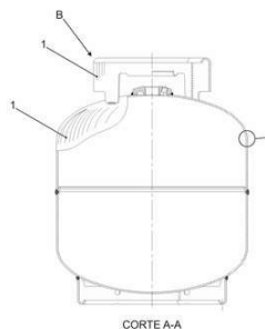
CORTE A-A
