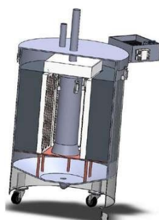
FIGURA 1. Representação completa do reator pirolítico.
