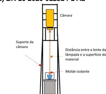
FIGURA 1 - Representação esquemática do funcionamento do sistema de monitoramento
