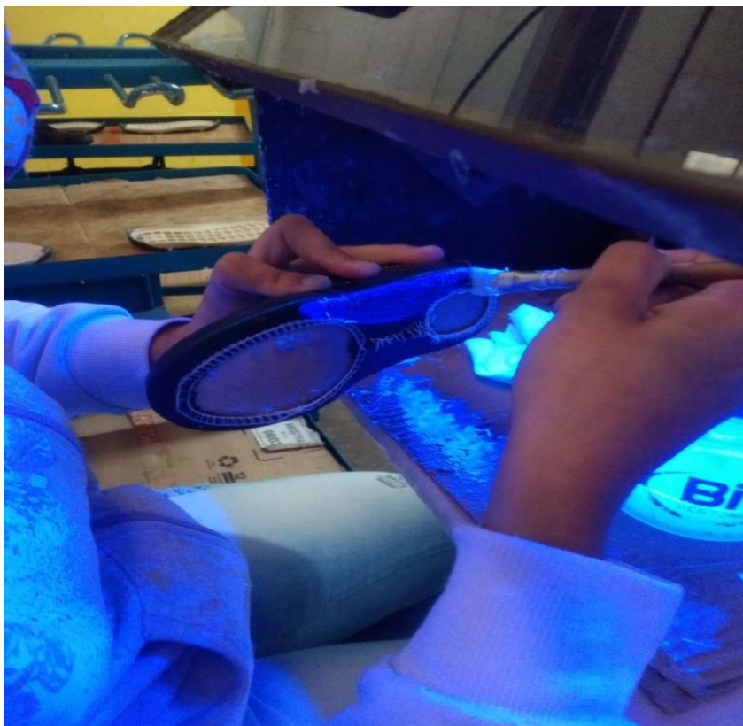
Foto 15 – Operação de unir solado ao cabedal.
