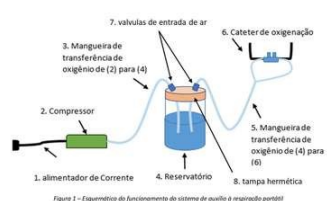
Figura 1 - Esquema de funcionamento do sistema de oxigênio portátil
