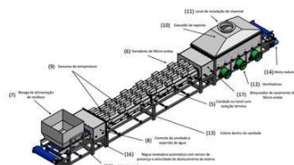
Figura 2 - A UNIDADE DE TRATAMENTO TÉRMIO (UTT) A MICRO-ONDAS PARA INATIVAÇÃO DE RESÍDUOS CONTAMINADOS MICROBIOLOGICAMENTE – Cavidade com acessórios.
