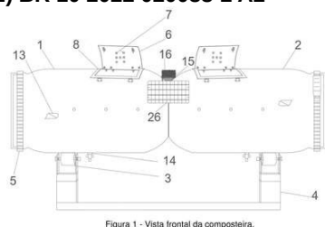
Figura 1 - Vista frontal da composteira.
