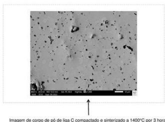
Imagem de corpo de pó de liga C compactado e sinterizado a 1400°C por 3 horas
