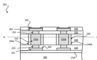
VISTA DE PERFIL EM SEÇÃO TRANSVERSAL
