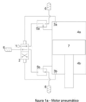
figura 1a - Motor pneumático
