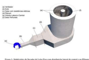
Figura 1 - Subdivisões do Secador de Leito Fixo com distribuição lateral de ar central e no Plenum
