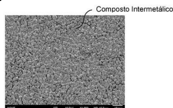
Composto Intermetálico
