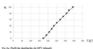
Fig 2a: Perfil de destilação do HP1 (diesel).
